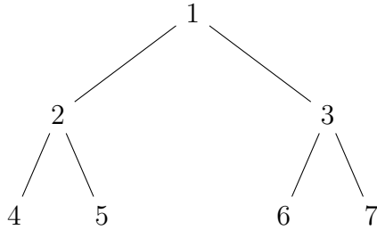
Albero binario completo
